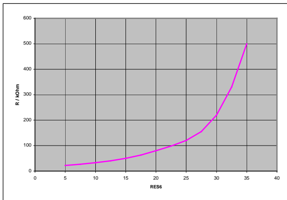
Bild 2: R / k\Omega = f ( RES / 6\text{Bit} )
