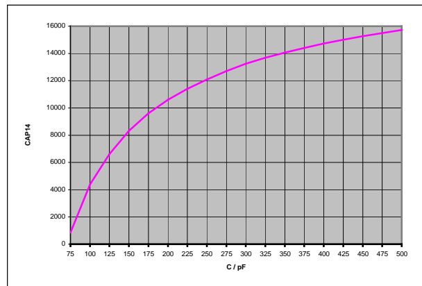
Bild 3: CAP / 14\text{Bit} = f ( C / pF )
