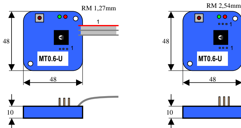
Bild 4: Abmessungen
